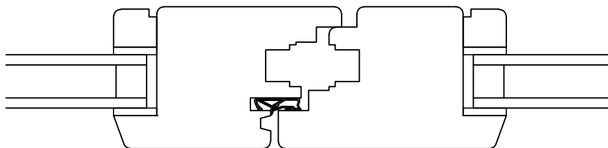
Naar Binnen Draaiend Raamstel Draai Kiep
