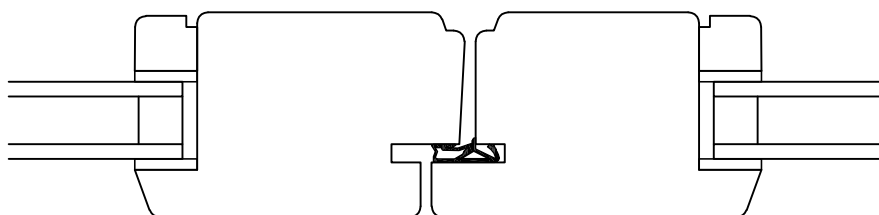
Naar Binnen Draaiend Raamstel
